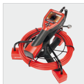
Modul 25/16 Duljina kabl/radni doseg: 16 m Radni prostor: do Ø 100 mm
