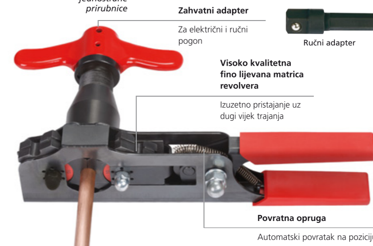
D-kontura jednostrane prirubnice
